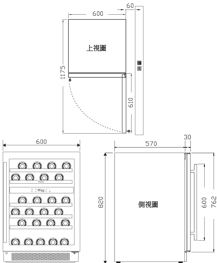
櫥下式紅酒櫃 預留空間尺寸圖
