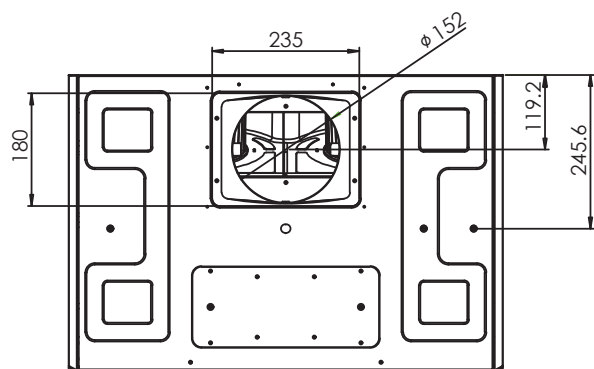
上視圖
