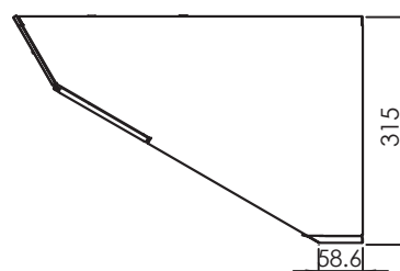
側視圖
